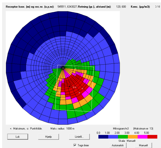
Figur 2: Lugtblastningen i afstande op til 1000 meter.
