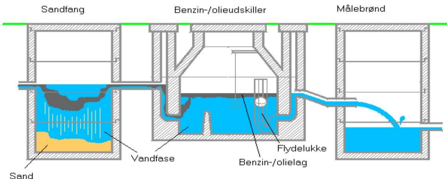
Principskitse af et olieudskilleranlæg med sandfang og målebrønd.
