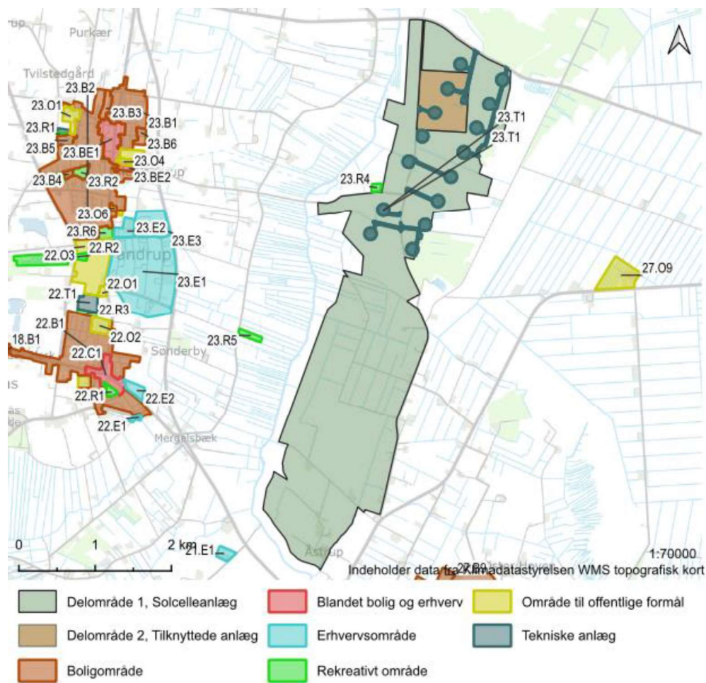
Figur 3-2 Gældende kommuneplanrammer inden for og nær energiparkens areal, bestående af delområde 1 og 2.
