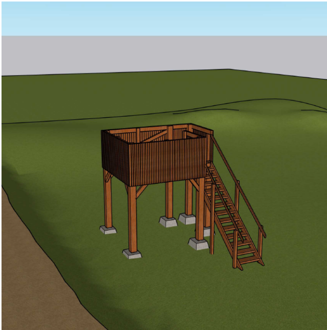
Bilag 2: Tegning og materialebeskrivelse af tårn
