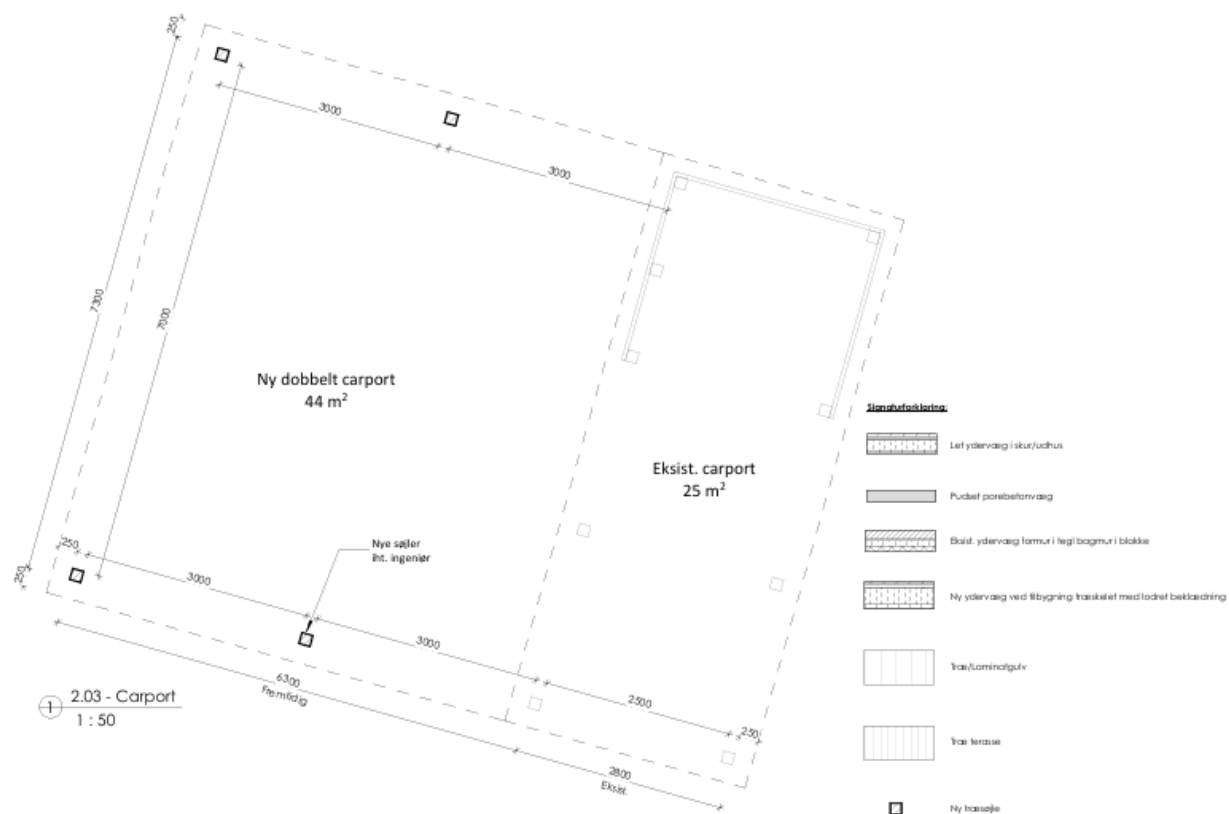
Figur 5: Carport - ikke målfast
