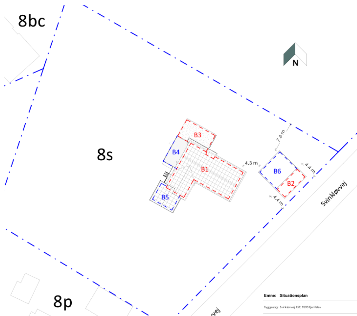
Figur 4: Situationsplan - eksisterende carport er markeret med B2, tilbygning er markeret med B6 - ikke målfast.
