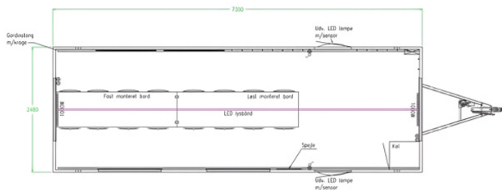
Figur 5: Specifikationer på kontorvognen - ikke målfast
