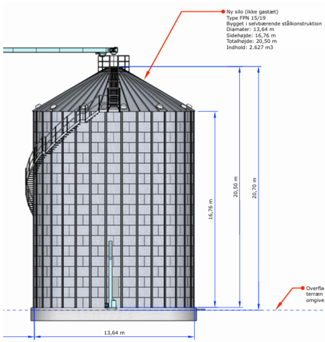
Figur 5: Silo mål og afstande
