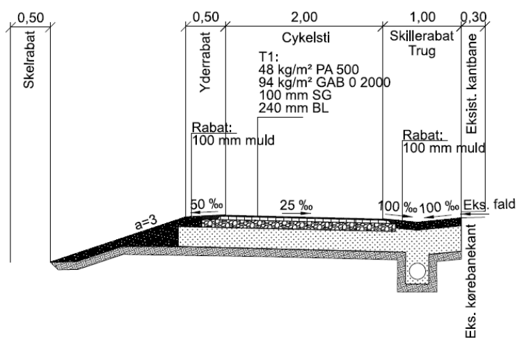
Figur 2. Tværsnit af cykelsti. Fra ansøgningsmaterialet.
